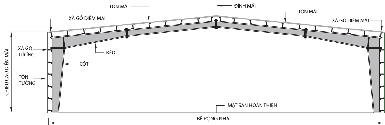
Mặt Cắt Ngang Điển Hình
