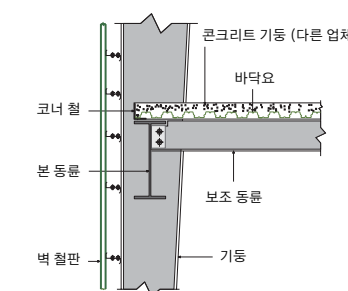
본 동륜과 보조 동륜 연결
