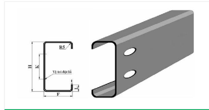
C 도리
