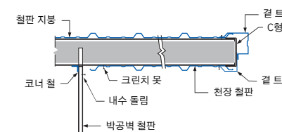
케노피 베란다와 천장 철판
