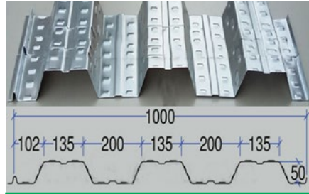
Decking 바닥 H=50
