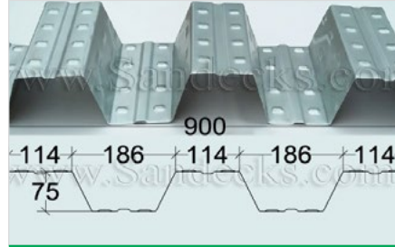
Decking 바닥 H=75
