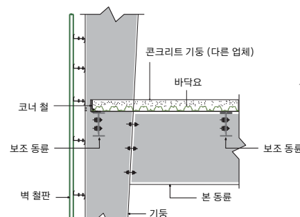
본 동륜과 본 기둥 연결
