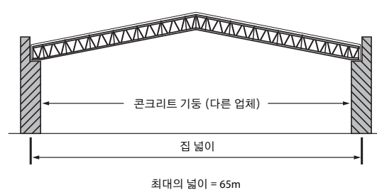
지붕 구조
