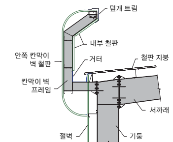
곡선 칸막이 벽
