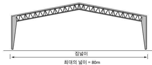
서까래
