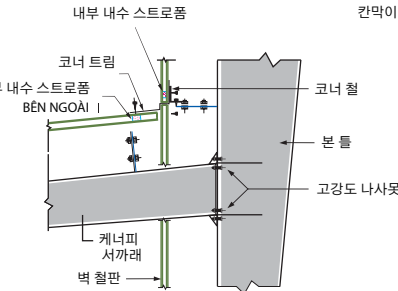
본 동륜과 보조 동륜 연결
