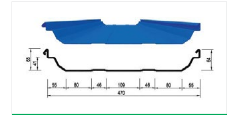
Seamlok 패널 프로파일
