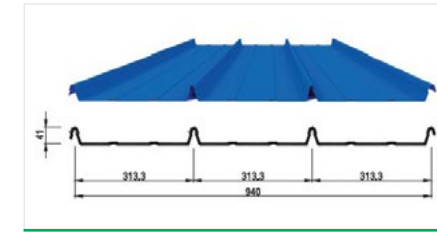
Kliplock 패널 프로파일
