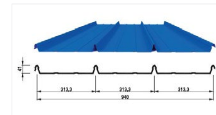
Kliplock波纹板
