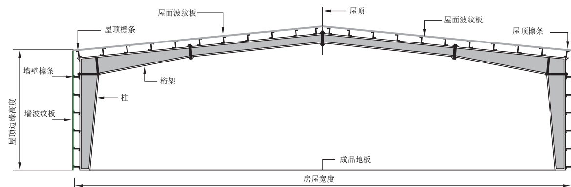
典型截面
