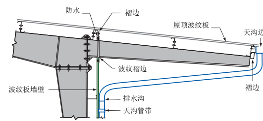
侧壁檐
