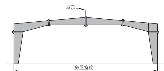
无中柱厂房
