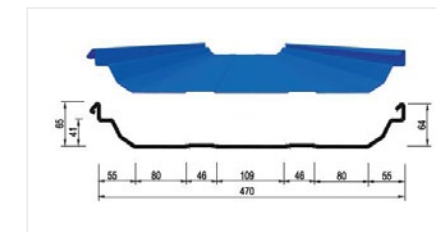
Seamlok波纹板
