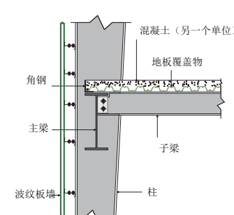
辅梁和主梁链接
