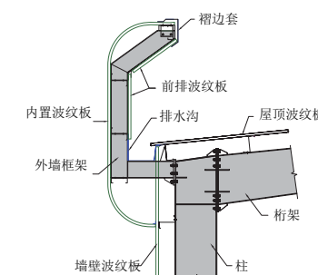
弯曲的门面
