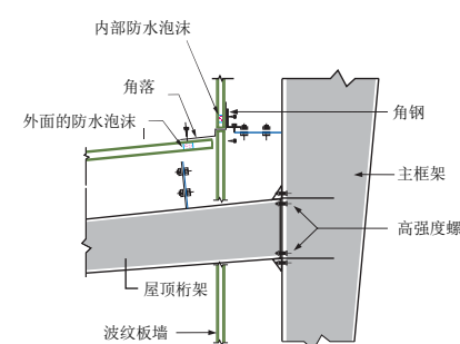
接合屋顶
