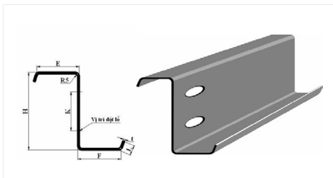
檩条 Z
