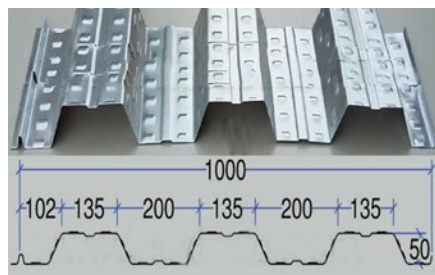
地板H = 50
