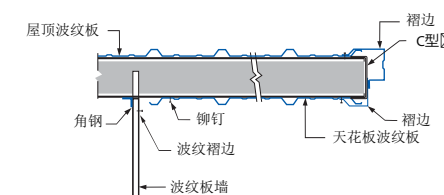
波纹板天花板遮阳篷
