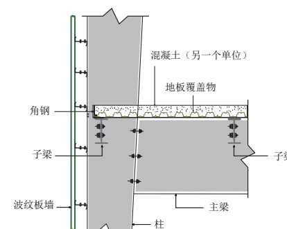
将主楼大梁链接到主框架列
