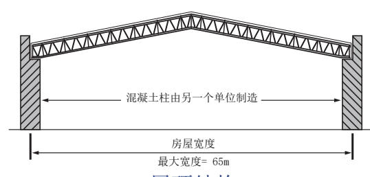
屋顶结构
