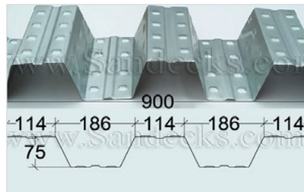
地板H = 75
