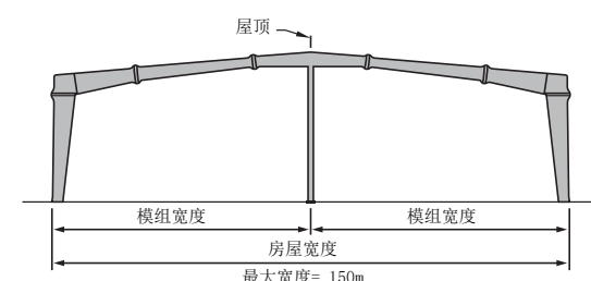
一个中柱房子
