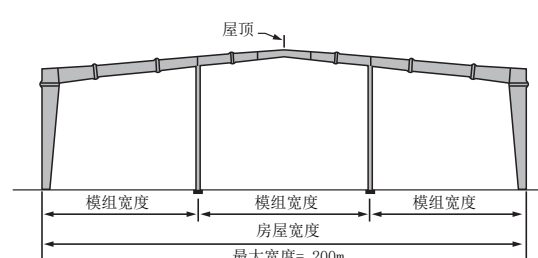
两个中柱房
