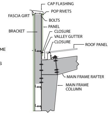
Parapet Fascia
